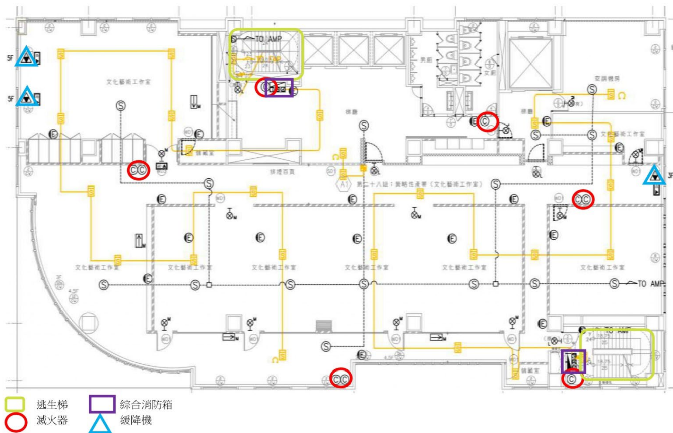
5樓 消防安全設備平面圖
